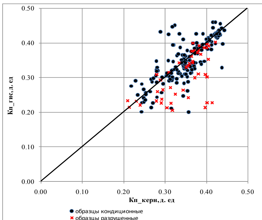
Рисунок 1 – Сопоставление коэффициентов пористости, определенных по керну и ГИС
