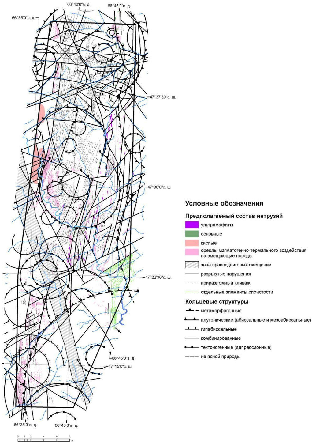
Рисунок 1 – Космоструктурная схема участка Карсақпай 1 : 200 000 масштаба
