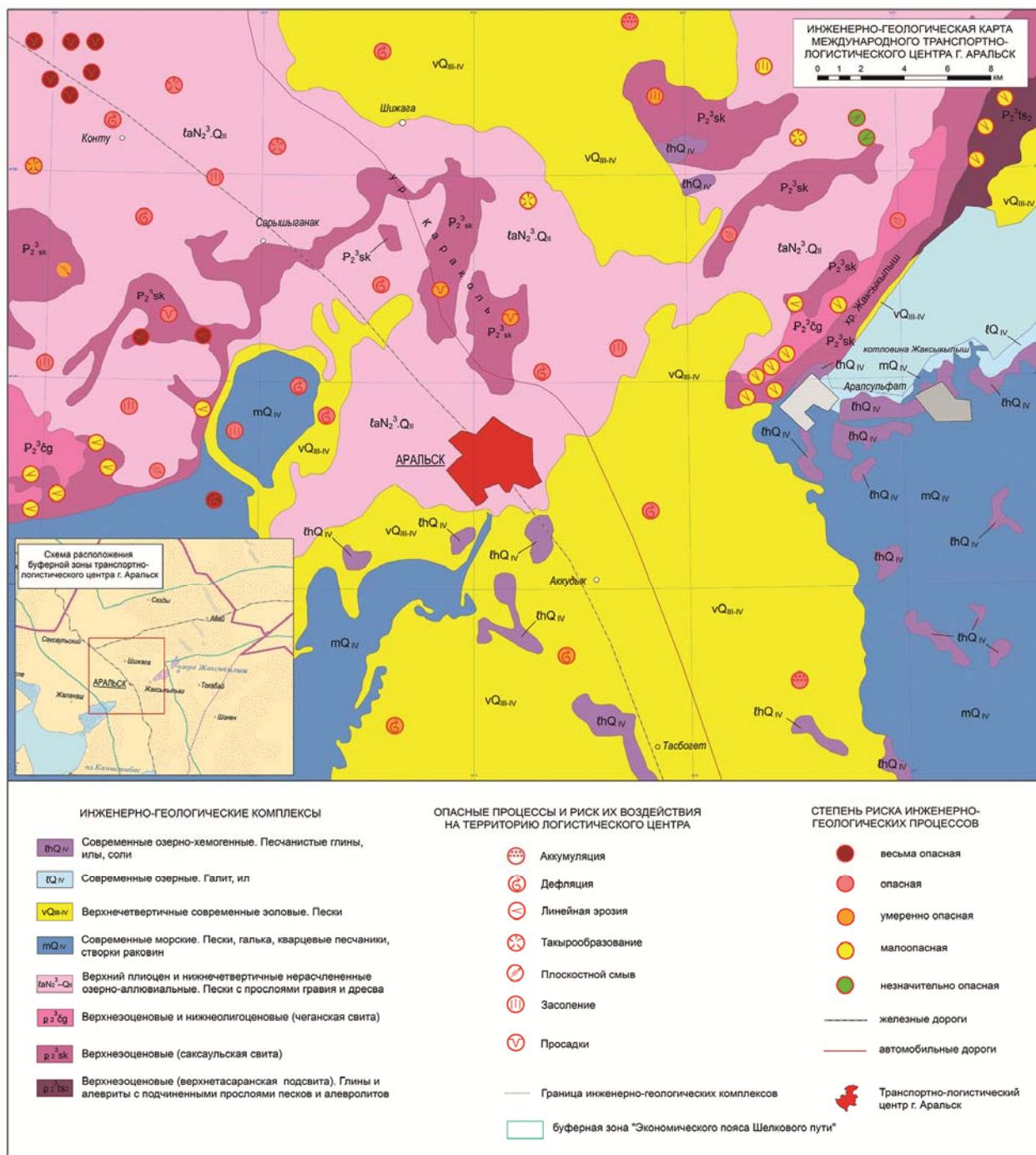
Рисунок 1 – Инженерно-геологическая карта международного транспортно-логистического центра г. Аральск
