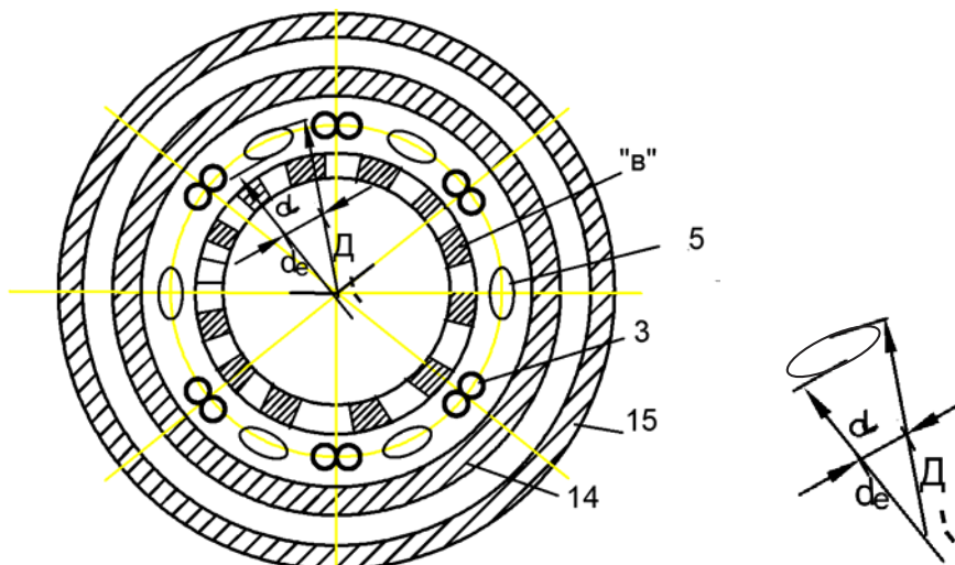
Рисунок 2 – Поперечный разрез экспериментального стенда по А-А (на рисунке 1)
