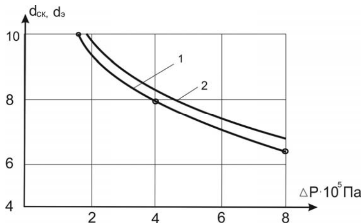
Рисунок 4 – Зависимость диаметра d_{\text{ск}} круглого сопла и щелевого сопла эквивалентного диаметра d_{\text{э}} от перепада давления \Delta P при прокачивании жидкости через кольцевой эжектор с постоянным расходом Q = 7 \text{ л/с} : 1 – кривая для круглого сопла диаметром d_{\text{ск}} ; 2 – кривая для щелевого сопла с эквивалентным диаметром d_{\text{э}}
