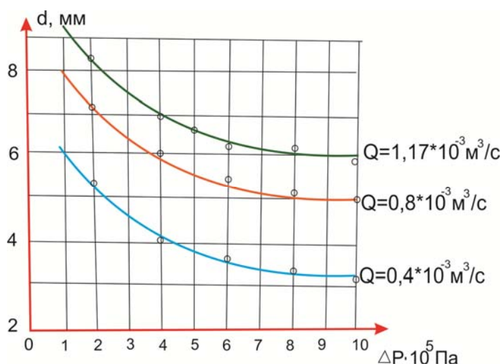
Рисунок 3 – Зависимость диаметра сопла d_{ск} от перепада давления в кольцевом эжекторе при различных расходах Q_p рабочего потока
