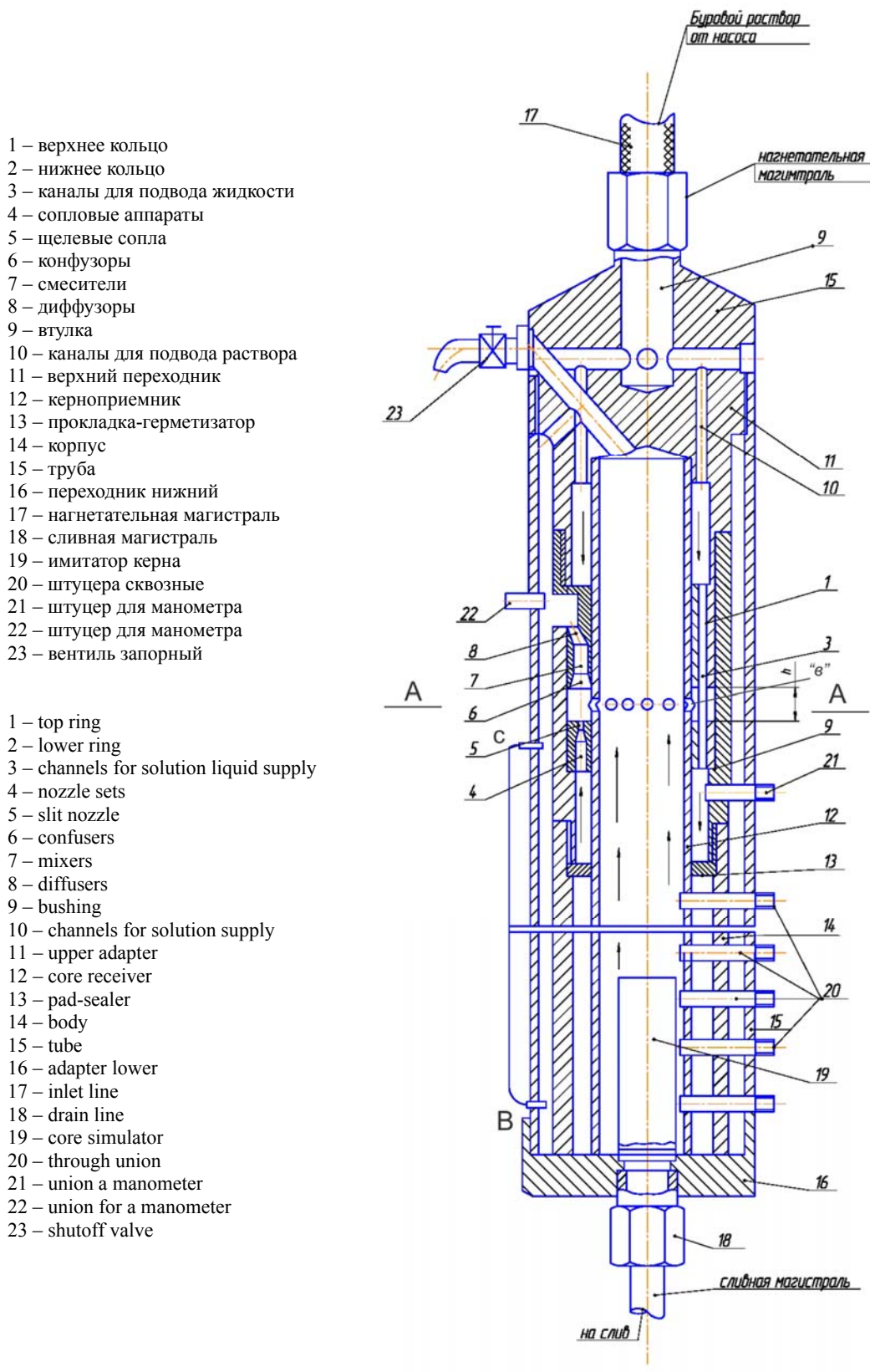
Рисунок 1 – Экспериментальный стенд для исследования параметров кольцевого эжектора (разрез COB на рисунке 2)
