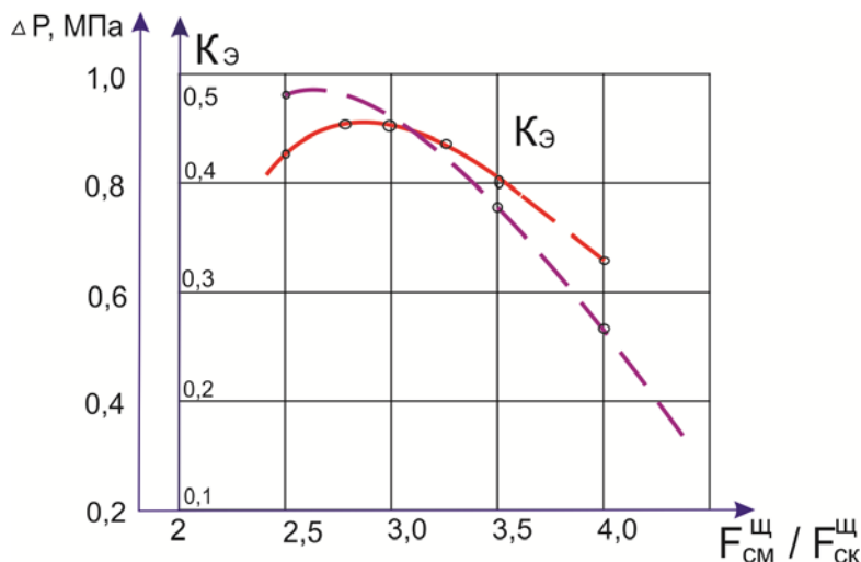
Рисунок 5 – Зависимость коэффициента эжекции K_{э} и перепада давления \Delta P_{см} в приемной камере от соотношения F_{см}^{щ}/F_{ск}^{щ} (эквивалентный диаметр щелевого сопла d_e = 10 мм)
