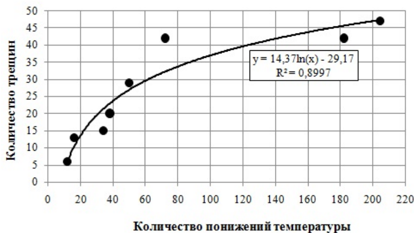
Рисунок 5 – Зависимость среднего количества температурных трещин на асфальтобетонном покрытии автомобильной дороги «Астана-Бурабай» от числа критических понижений температуры воздуха
