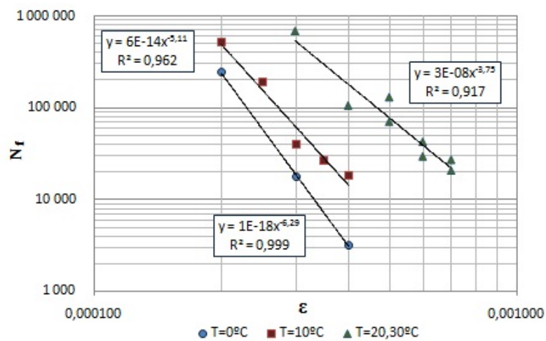
Рисунок 4 – Зависимость усталостной прочности асфальтобетона от деформации при разных температурах
