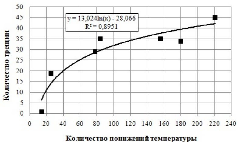
Рисунок 6 – Зависимость среднего количества температурных трещин на асфальтобетонных покрытиях автомобильных дорог, расположенных в Акмолинской, Акт'yбинской, Алматинской, Костанайской и Кызылординской областях, от числа критических понижений температуры воздуха
