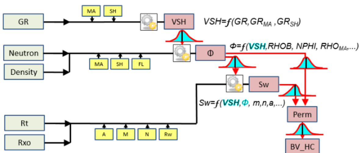
Рисунок 5 – Схема обработки диаграмм ГИС
