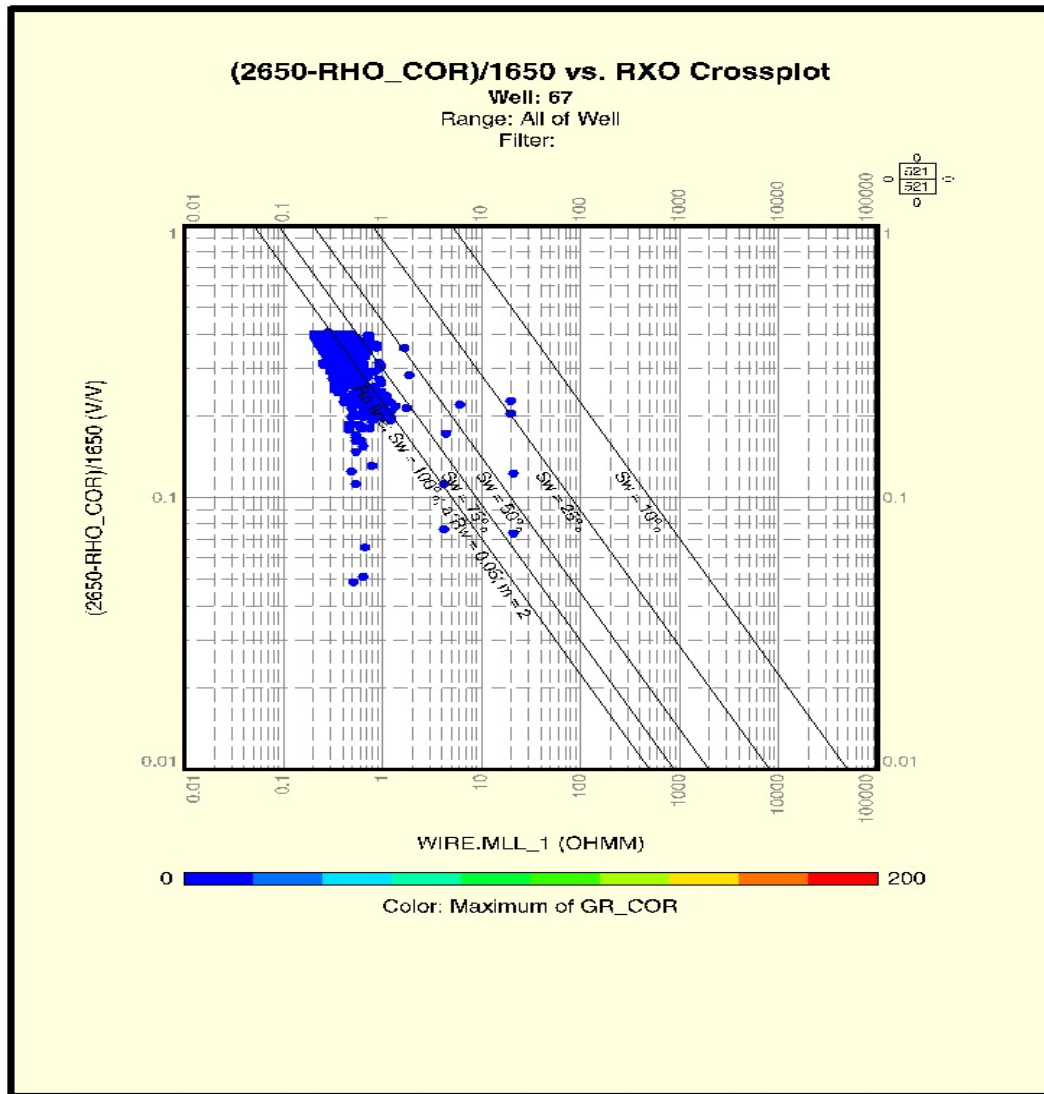
Рисунок 8 – Определение характера насыщения пластов коллекторов по изучаемой скважине
