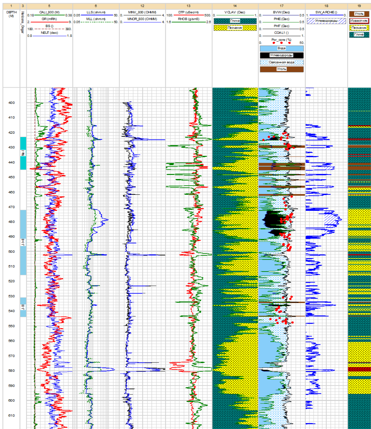
Рисунок 1 – Изучение разреза скважины по комплексу ГИС
