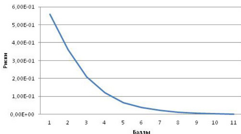
Рисунок 6 – Кривая сейсмической опасности для точки
